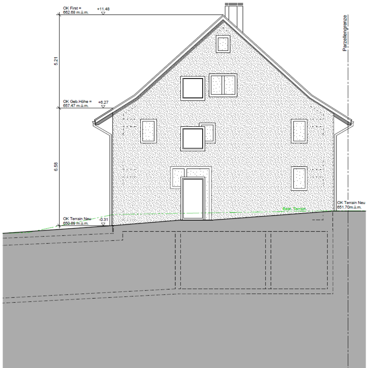
ANSICHT NORDFASSEDE
