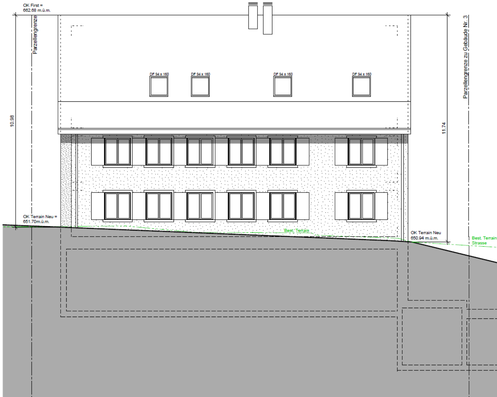
ANSICHT WESTFASSE
