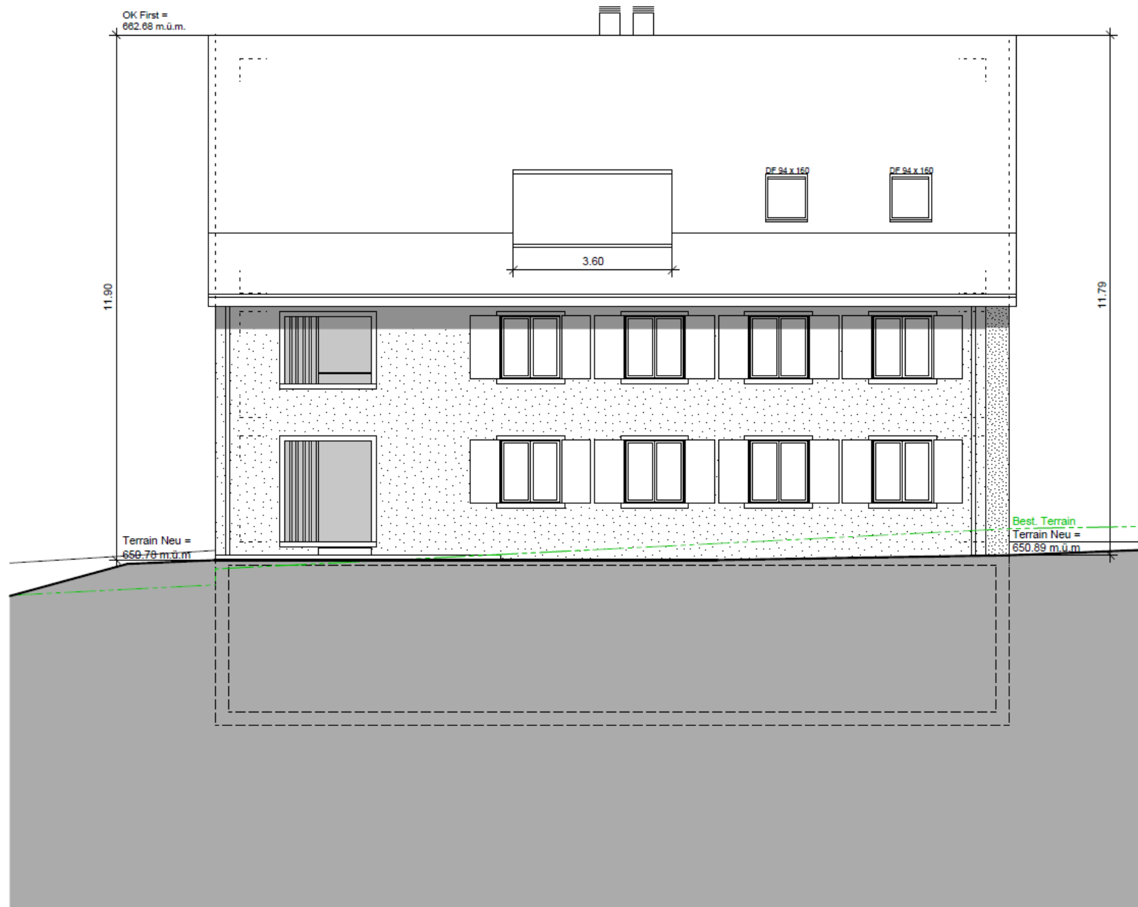
ANSICHT OSTFASSADE
