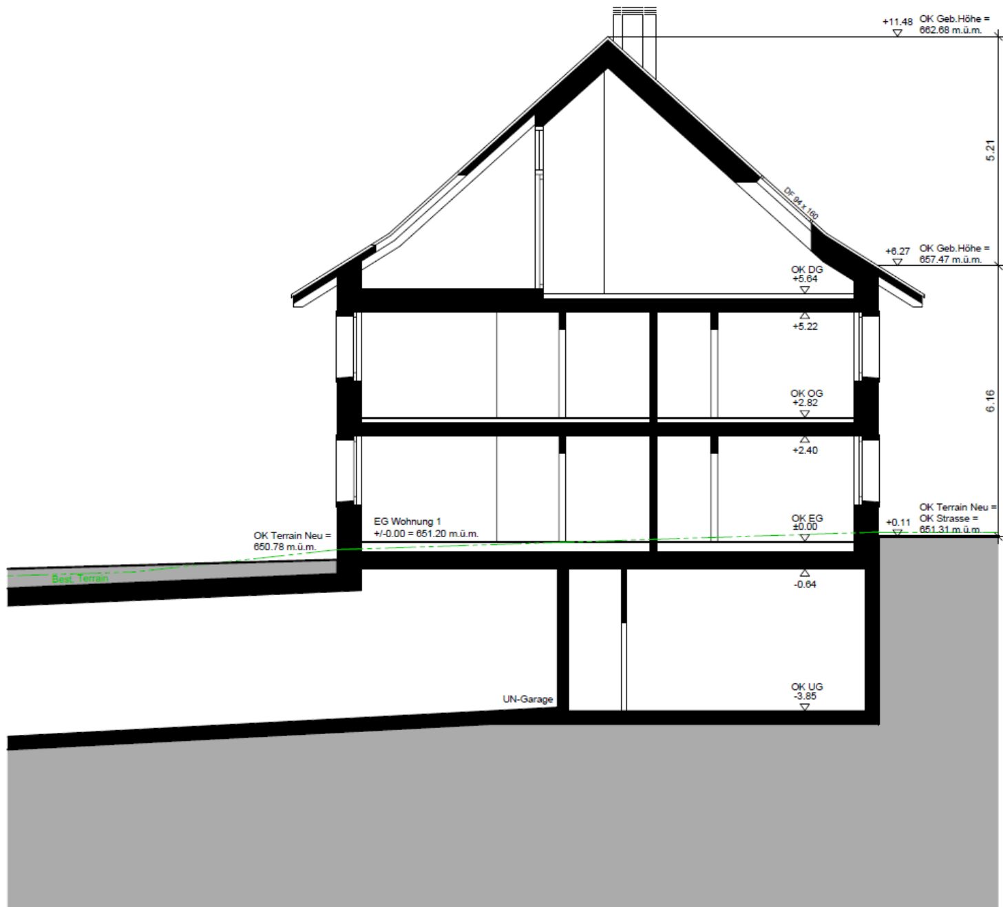
SCHNITT 2 - 2
