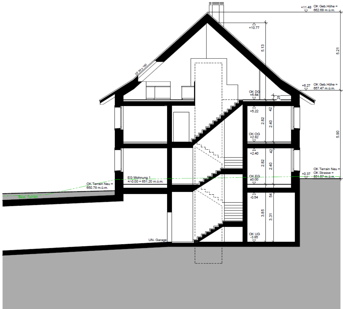
SCHNITT 1 - 1
